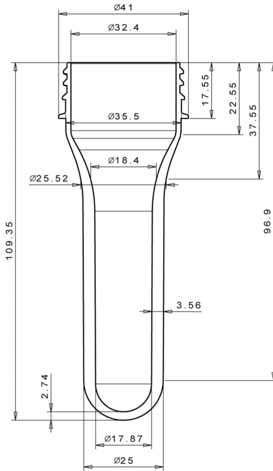
A-A View/görünüm
